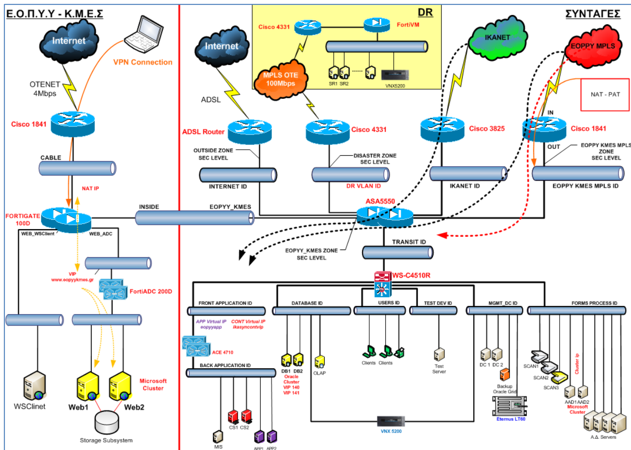
Σχήμα 2: Αρχιτεκτονική ΚΜΕΣ
